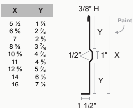
Fascia Trim
