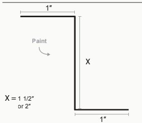
Z Bar
