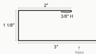
Soffit C Metal
