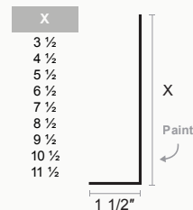
Open Jamb
