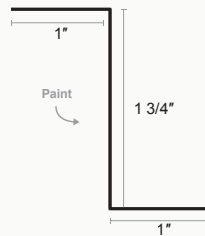
Z Bar_1.75
