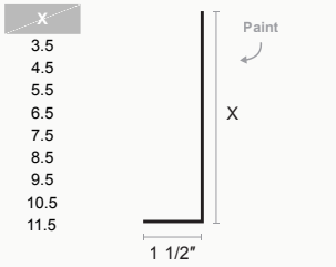
Open Jamb
