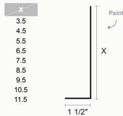
Open Jamb
