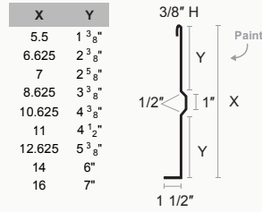
Fascia Trim
